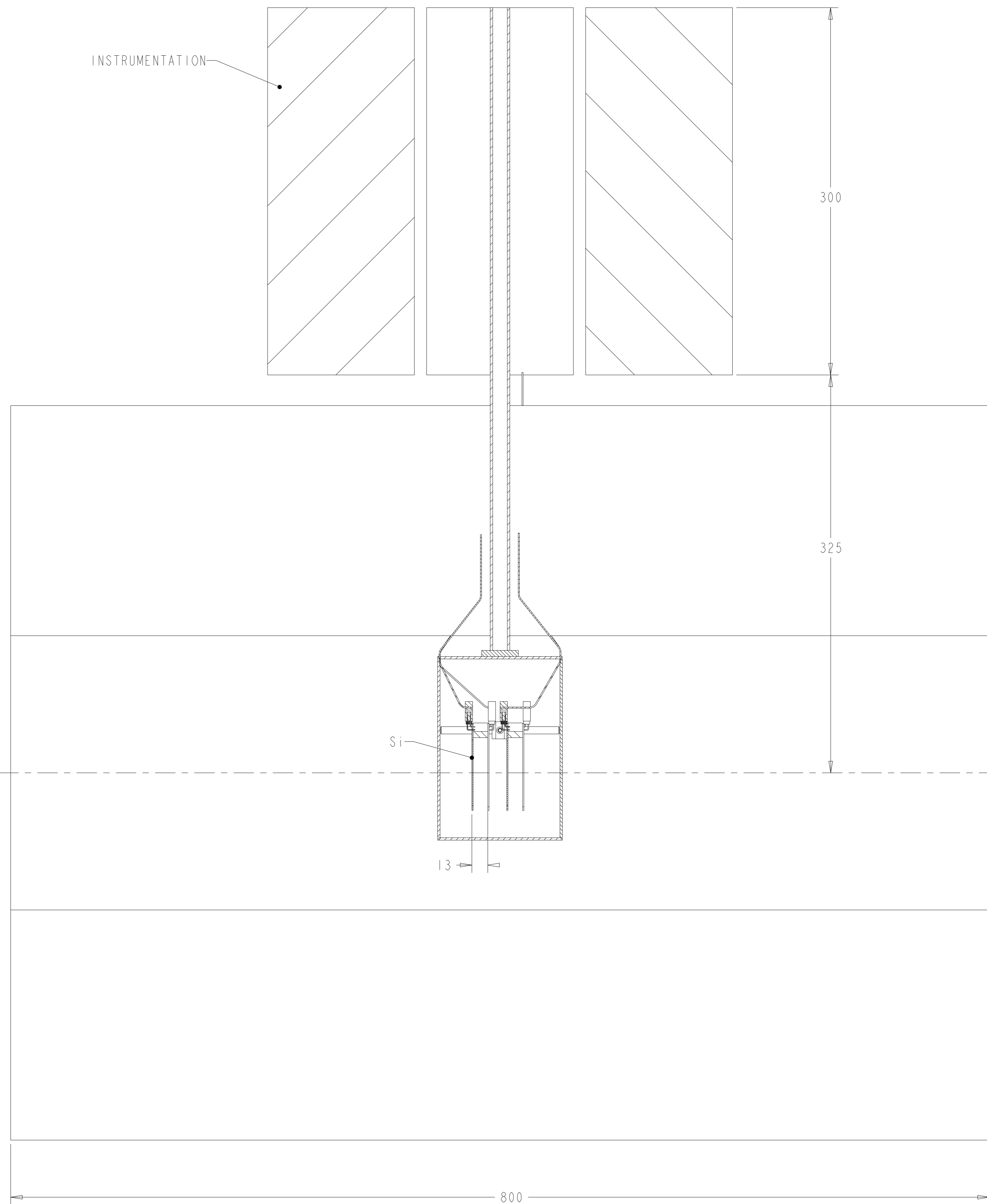
SECTION A-A
