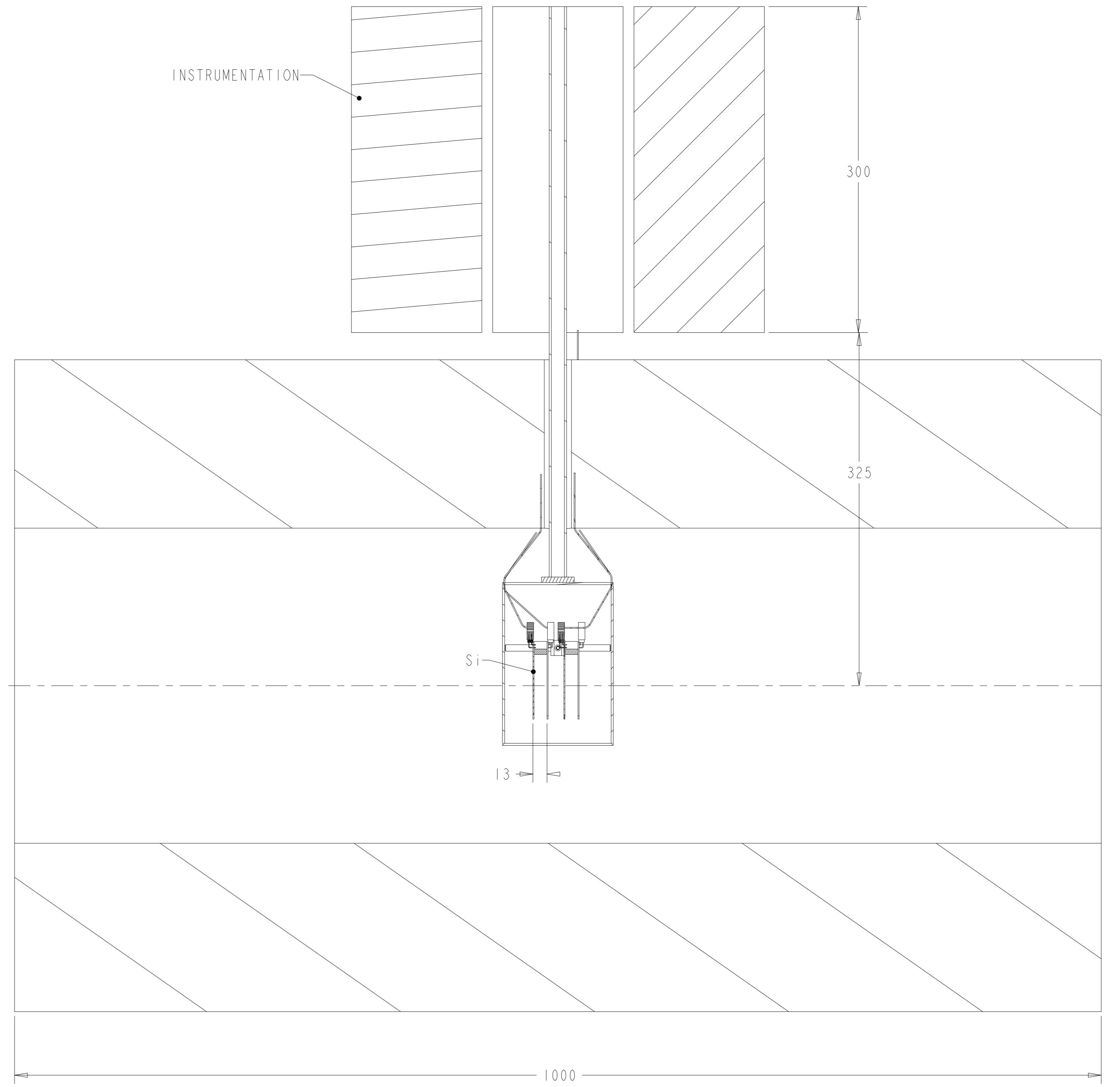
SECTION A-A
